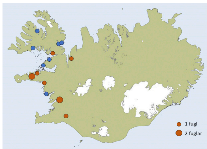
2. mynd. Dauðir eða vanfærir ernir sem fundust á Íslandi 1996–2020 og talið er að hafi flogið á raflínur. Rauðir hringir tákna fugla sem fundist hafa við línur Landsnets en bláir fugla sem fundist hafa við línur Rarik og Orkubús Vestfjarða.
